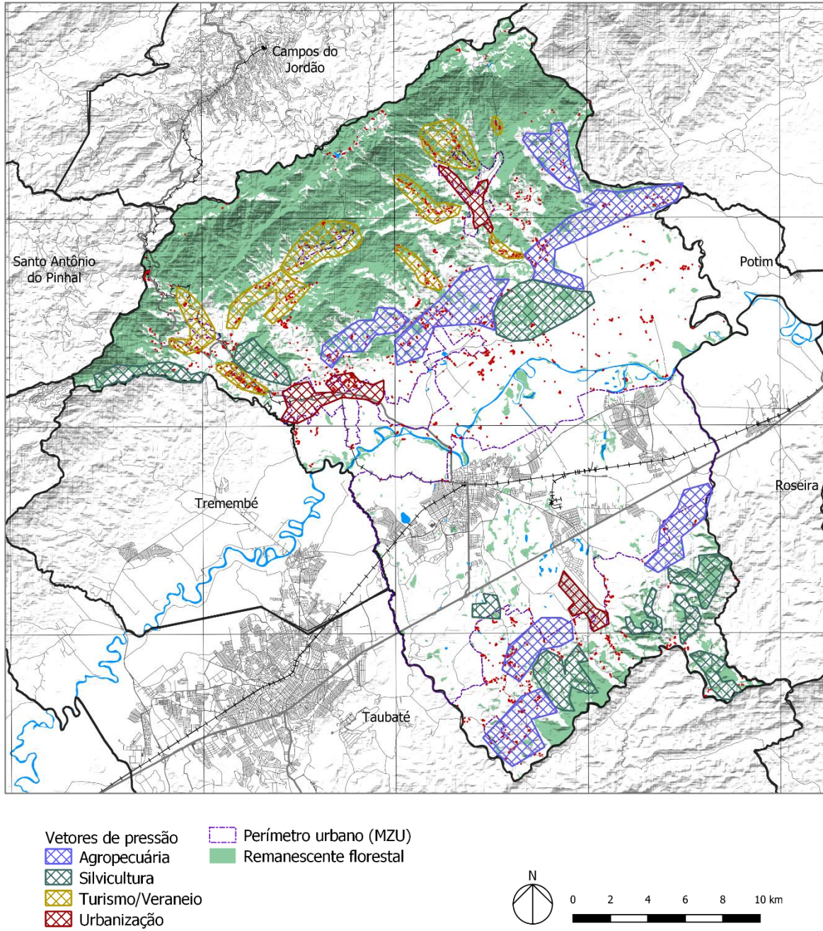
Figura 4-1 Mapa de vetores de pressão e desmatamento de Pindamonhangaba/SP
