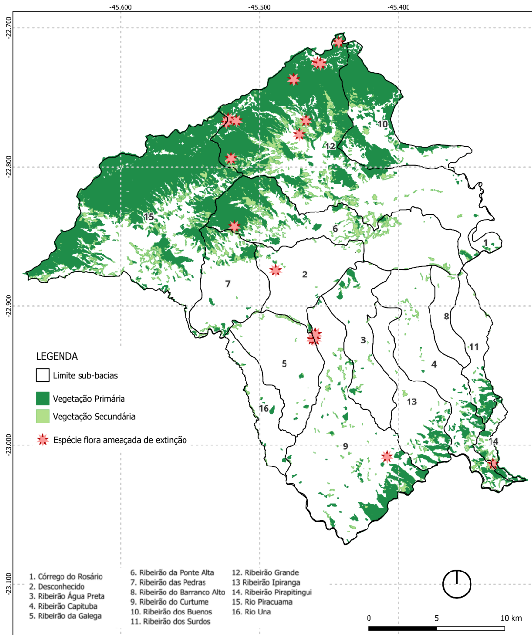
Figura 5-8 Espécies Ameaçadas de Extinção por Sub-bacia
